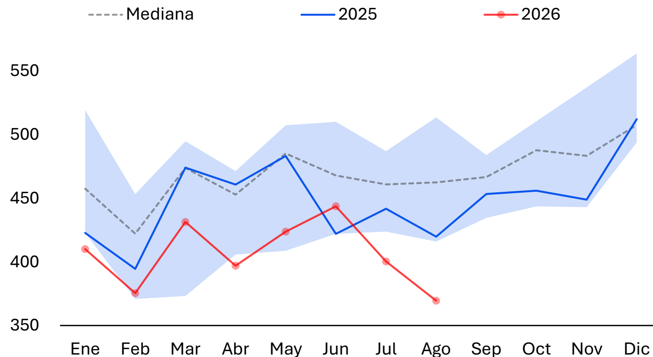
Producción mensual de cobre, Miles de Toneladas Métricas Finas. (banda: rango 2014–2025)
